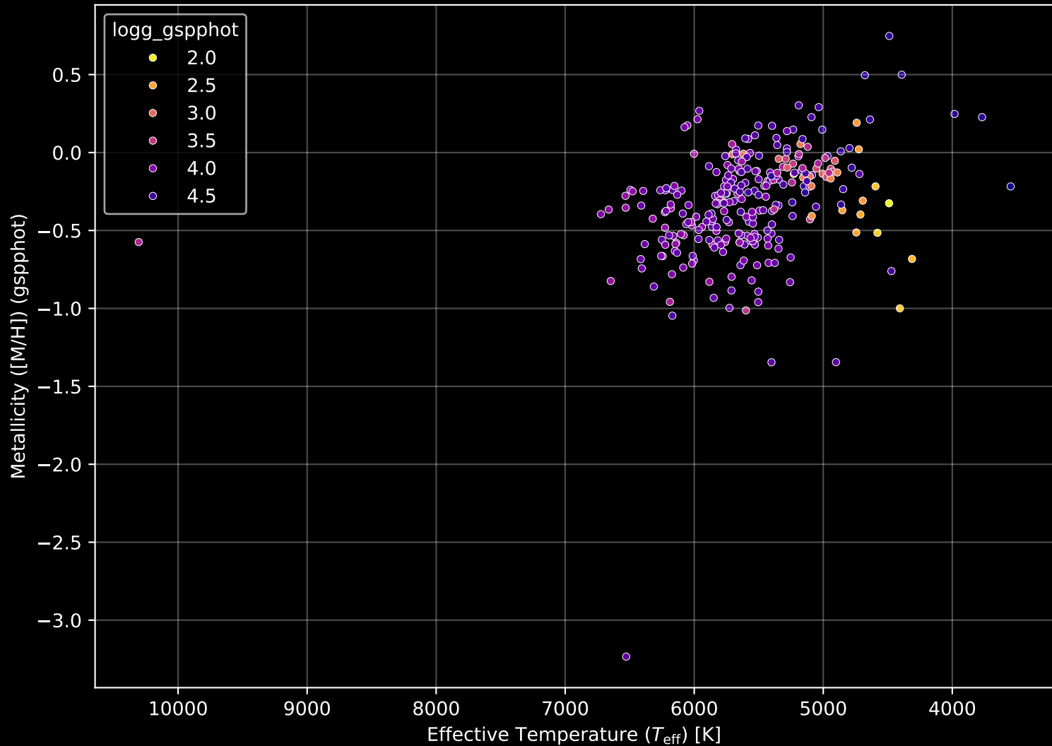
GALAH DR4 Field: [332] Stellar Population Parameters (n= 276)
