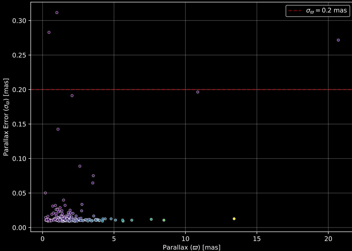
GALAH DR4 Field: [332] Parallax Quality (n= 276)
